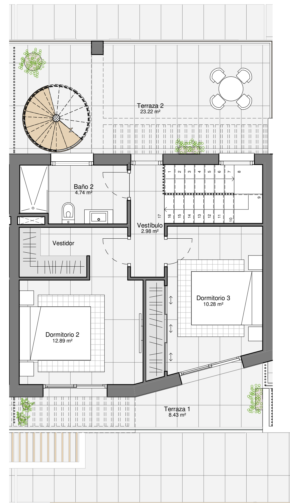
PRIMERA PLANTA / FIRST FLOOR
