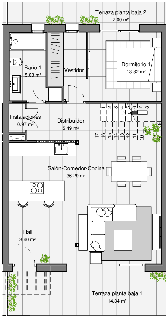
PLANTA BAJA
