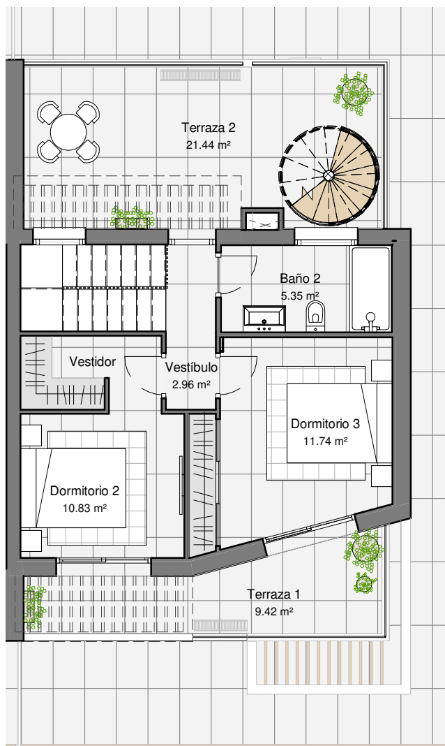
PLANTA PRIMERA
