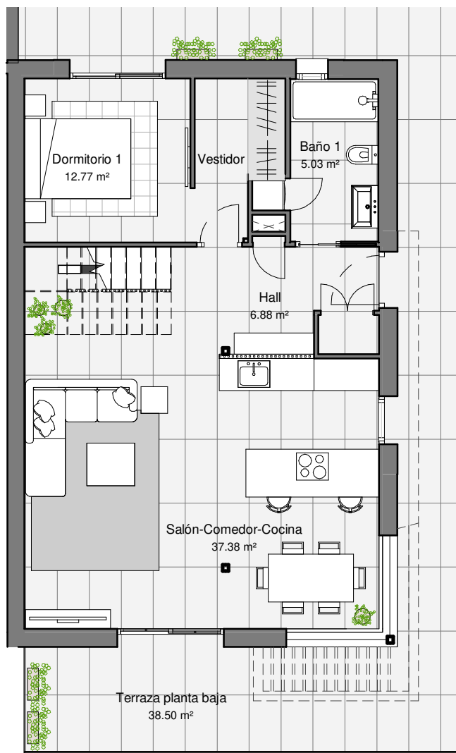
PLANTA BAJA
