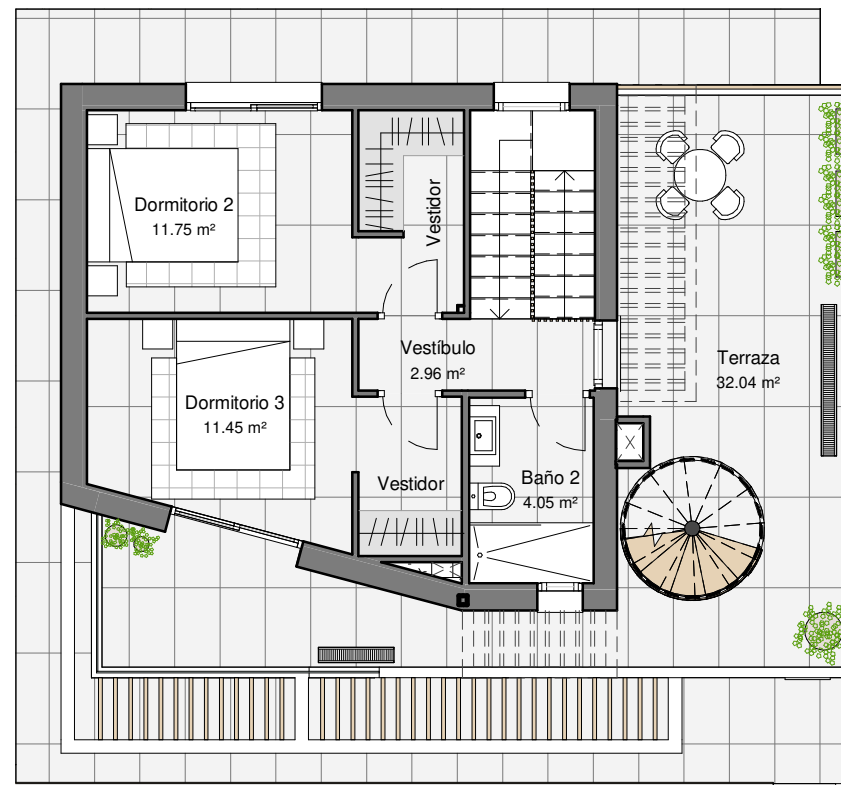
PLANTA PRIMERA
