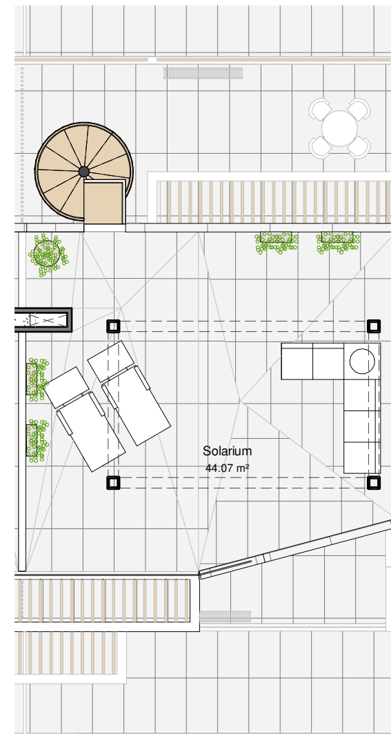
PLANTA CUBIERTA
