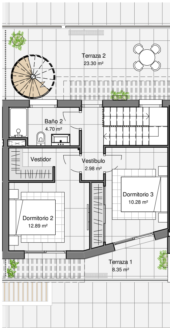
PLANTA PRIMERA
