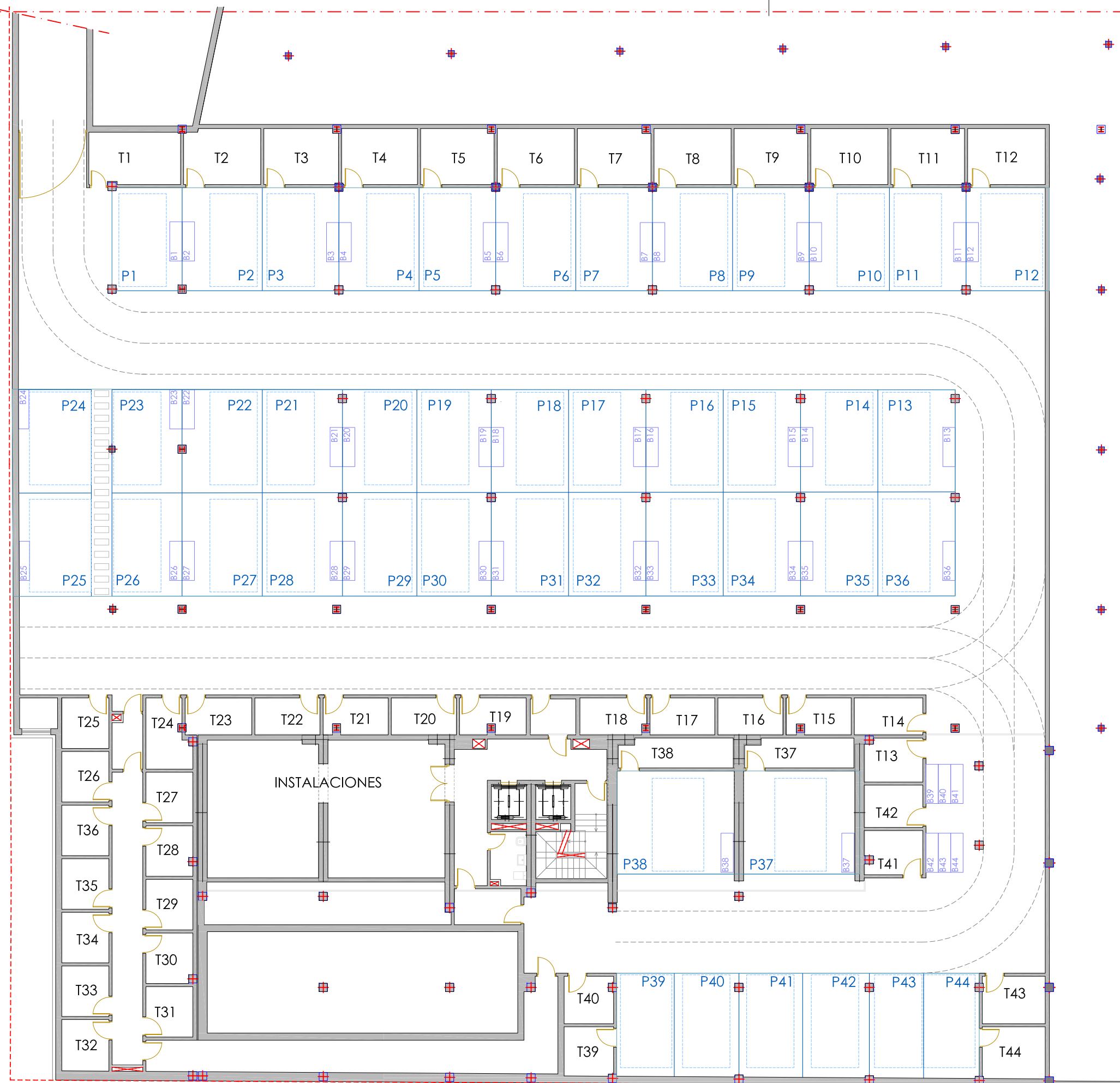
EDIFICIO DE 44 VIVIENDAS, GARAJE Y LOCALES SIN USO E 1/200
